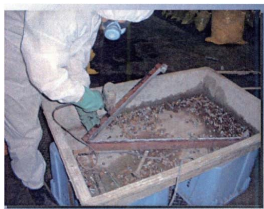
図4.10.7 掻き落とし除去作業の例
