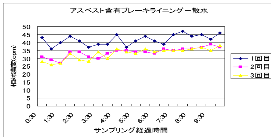
参考図 5.10 相対濃度計による粉じん濃度 (アスベスト含有ブレーキライニング散水状態)
