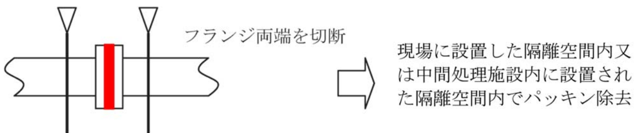
図4.10.10 配管用シートパッキン解体・撤去例
