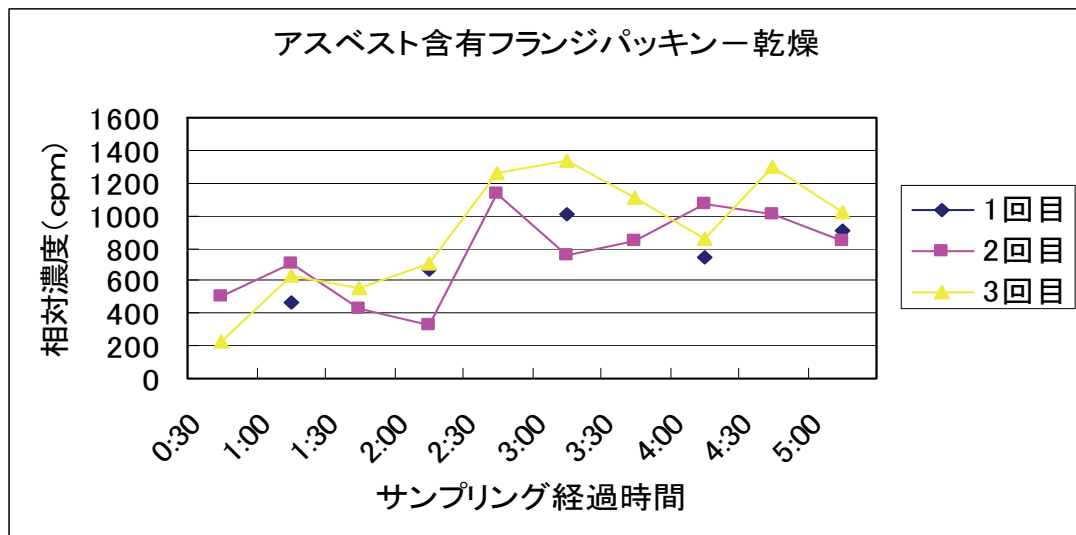
図7 相対濃度計による粉じん濃度（アスベストフランチパッキン乾燥状態）
