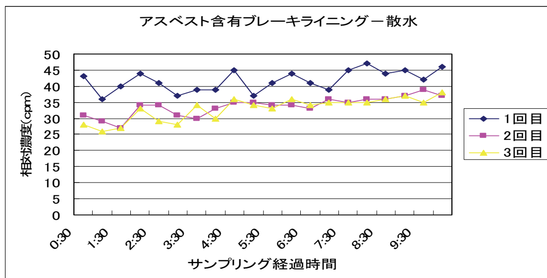
図10 相対濃度計による粉じん濃度 (アスベスト含有ブレーキライニング散水状態)
