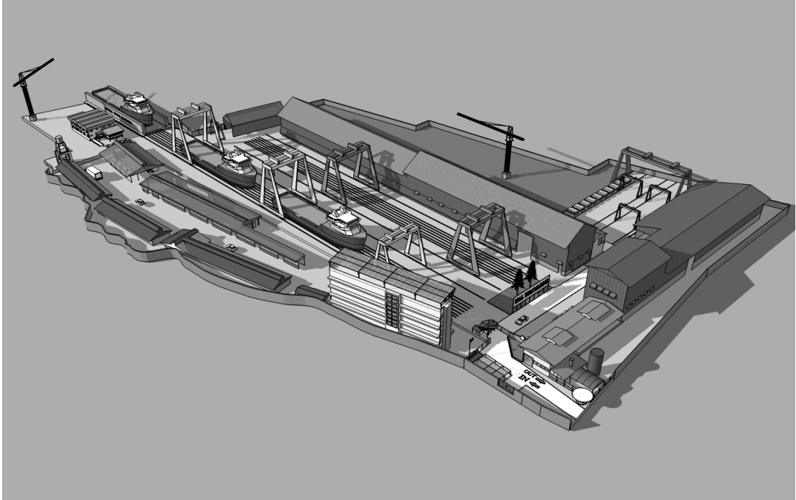
図 13 現在の造船設備
