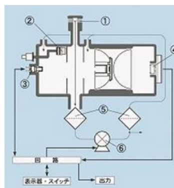
①採気口 ②散乱板 ③発光部 ④受光部 ⑤フィルタ ⑥吸引ポンプ 参考図4.3 粉じん相対濃度計の構造の例
