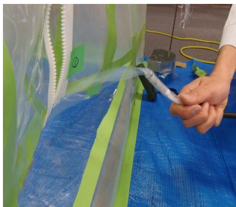
参考図4.10 スモークテスターによる確認
