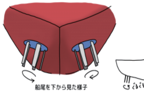
図 45 フォイトシュナイダープロペラ
