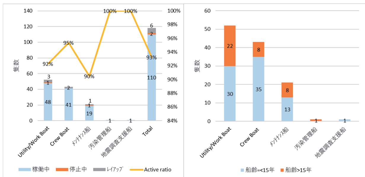
図 33 サウジアラビアのUtility Vesselの稼働率と船齢
