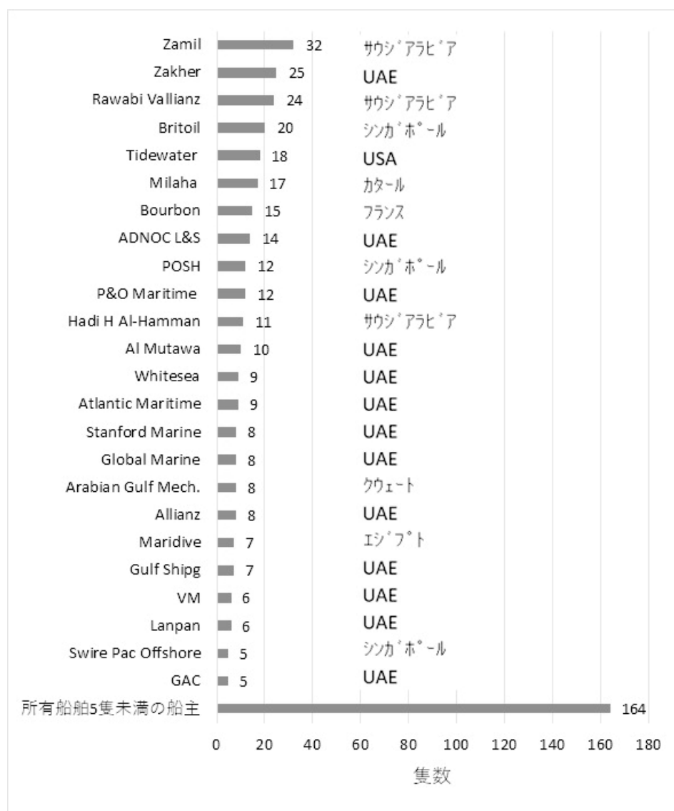
図 20 GCCのAHT/AHTS主要船主と所有隻数
